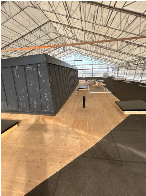
Nytt tak hus 44, ställning för ventilationsaggregat.
